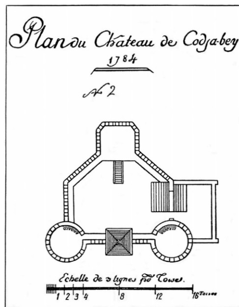
Рис. 2. План замка Коджа-Бей 1784 г. (Прил. П.3)
